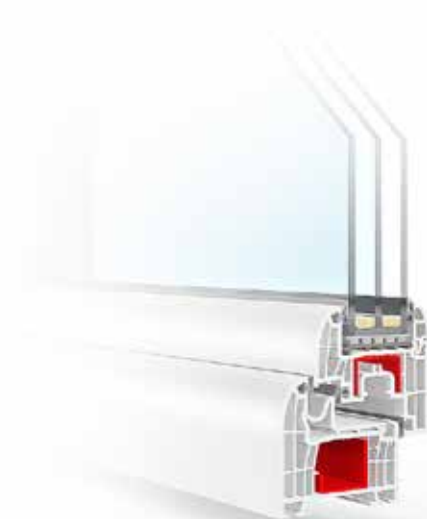
7 camere profondità telaio 70 mm
