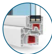
T-Energy 6 camere profondità telaio 88 mm
