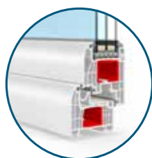
T-Passive Forte In/Out 5 camere profondità telaio 70 mm
